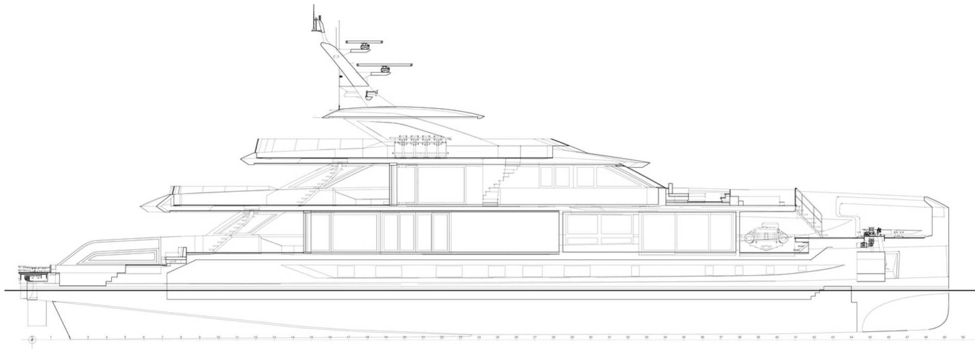
LONGITUDINAL SECTION
